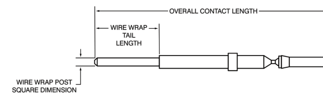
Wire Wrap Contact
